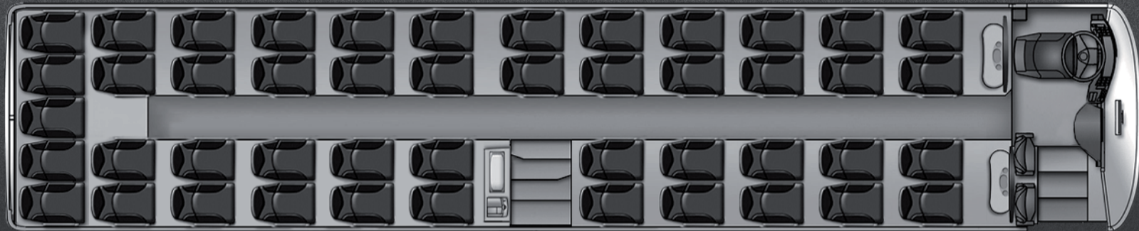
Floorplan Setra (49 +2 Sitzplätze)
